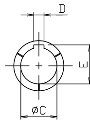
INPUT SHAFT
